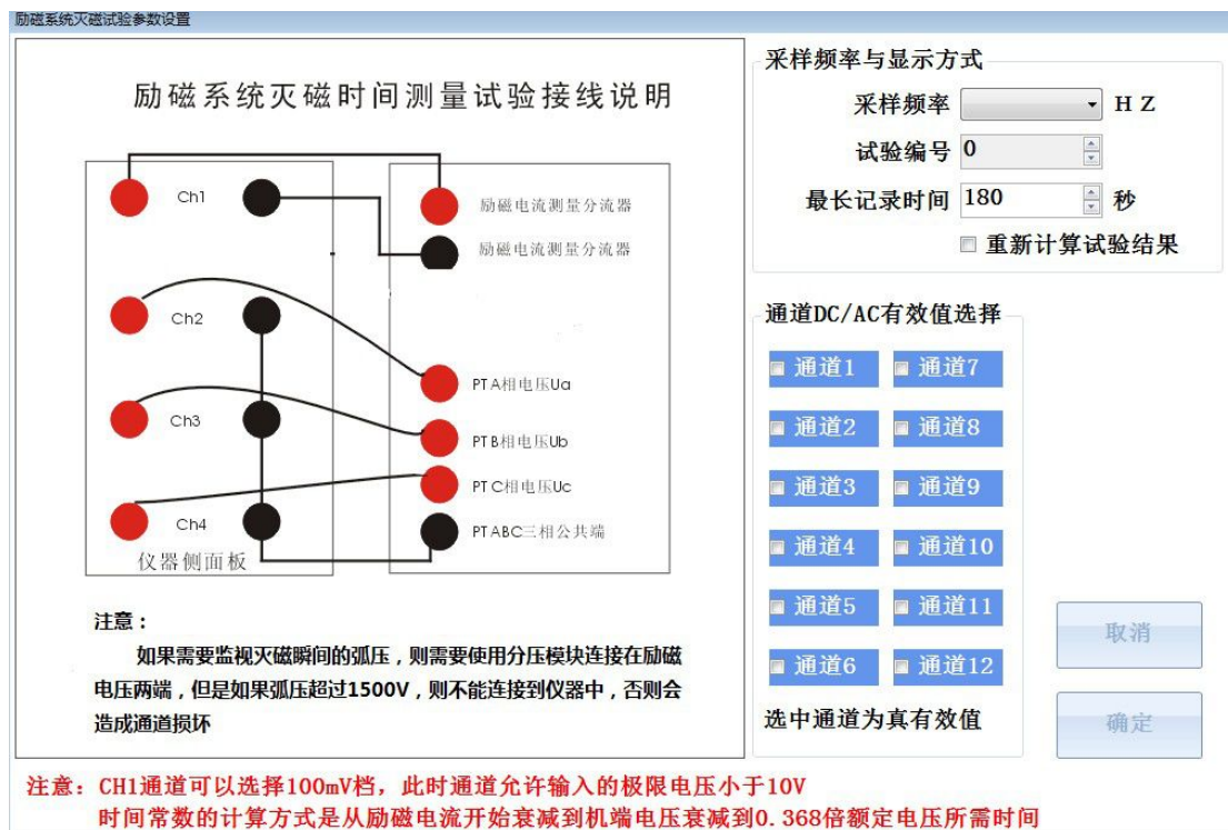
图 38 灭磁试验参数设置
