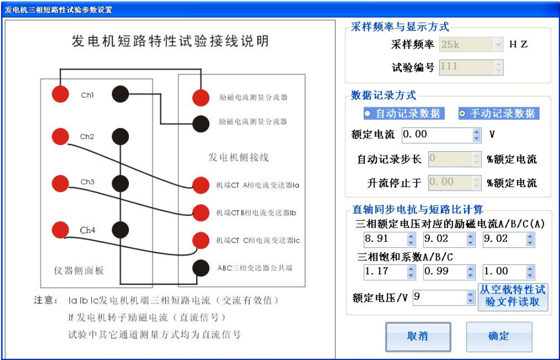
图 32 短路特性试验参数设置
